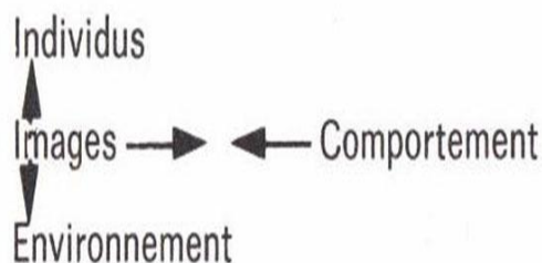
Figura 298. Schema di Wood (1970).
