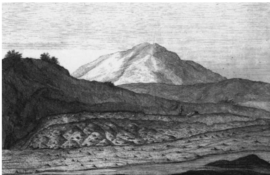
Figura 372. Le rive del fiume Mesima caratterizzate dalla comparsa di centinaia di vulcanelli dovuti al fenomeno della liquefazione delle sabbie. Fonte: Sarconi, 1784.
