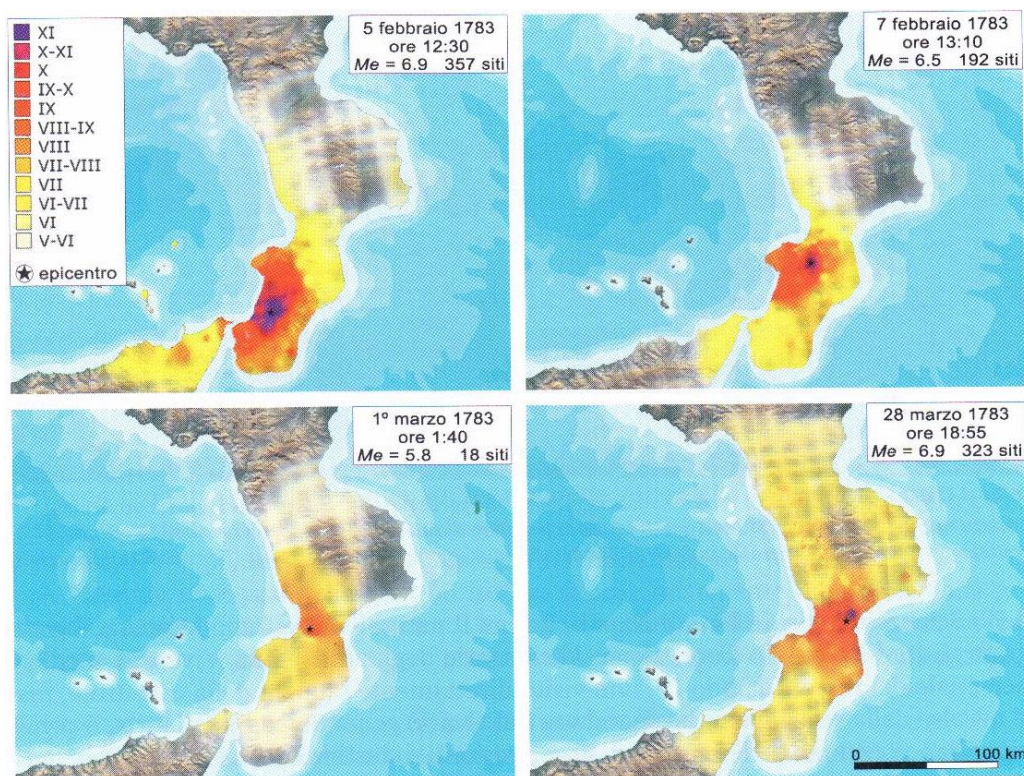
Figura 368. Localizzazione degli effetti dei terremoti del 5 e 7 febbraio, 1° e 28 marzo 1783. Le ore sono indicate in tempo universale (UT), che anticipa di un'ora rispetto all'ora locale (dati elaborati dal CFTI4Med). Fonte: Comastri, Mariotti, 2008.
