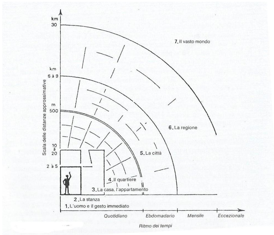
Figura 304. Le conchiglie dell'uomo secondo Moles e Rohmer. Fonte: Frémont, 1976, p. 24.
