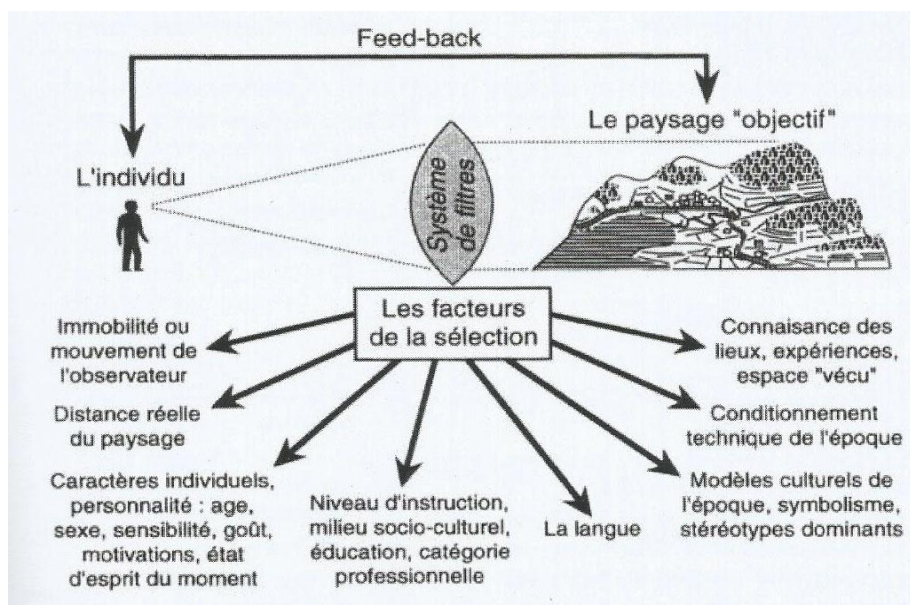
Figura 301. Lo schema concettuale della percezione dello spazio geografico di Roger Brunet, rivisitato da Jean Paulet. Fonte: Paulet, 2009.
