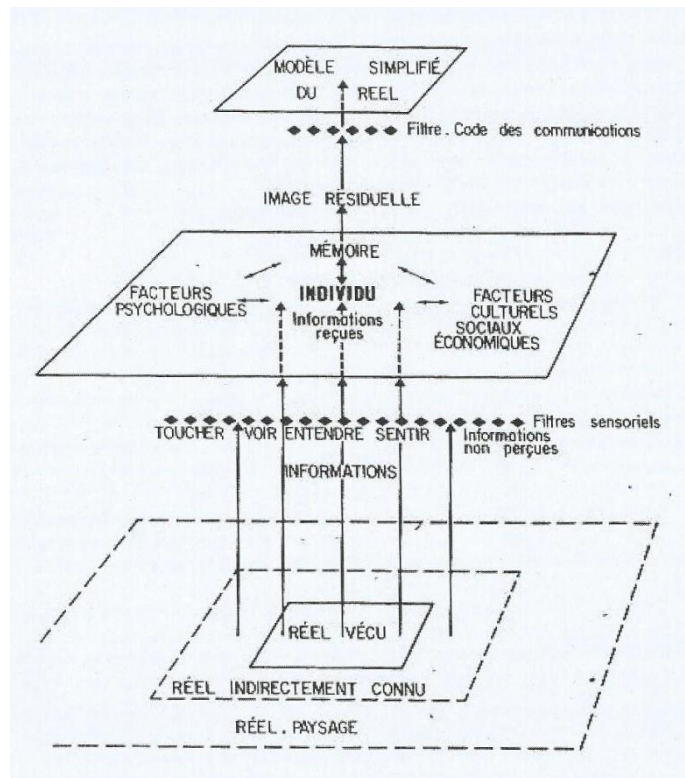
Figura 302. Lo schema concettuale della percezione dello spazio geografico di Antoine Bailly. Fonte: Bailly, 1975.
