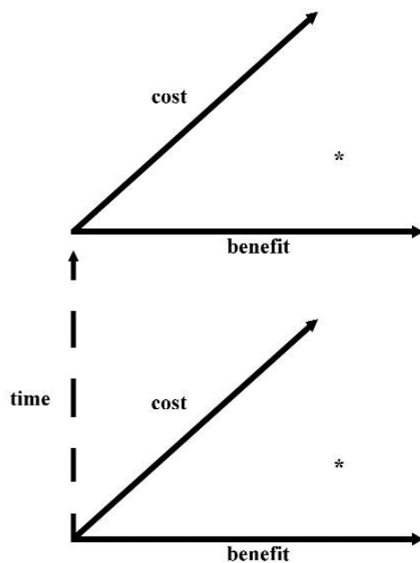
Figura 336. Rapporto costi-benefici a lungo termine nell'approccio geoetico. Fonte: Matteucci et al. , 2012.
