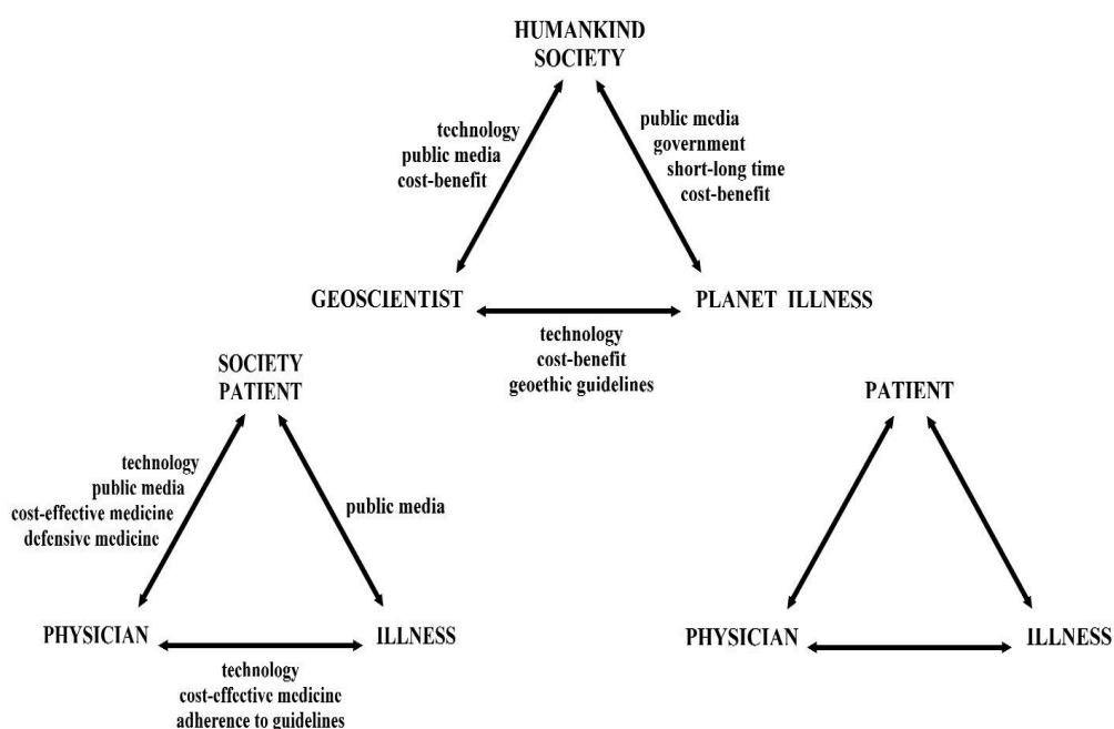
Figura 335. Fattori che influenzano il Triangolo Ippocratico [ispirato ad Antoniou et al. , 2010], in medicina (il medico, la malattia, il paziente / società) e nelle Scienze Geologiche (geoscientisti, 'malattia del Pianeta' - pericoli, impronta umana - e società). In basso a destra: le prime relazioni secondo Ippocrate. In basso a sinistra: nella medicina di oggi. In alto: l'equivalente dei geoscientisti. Fonte: Matteucci et al. , 2012.
