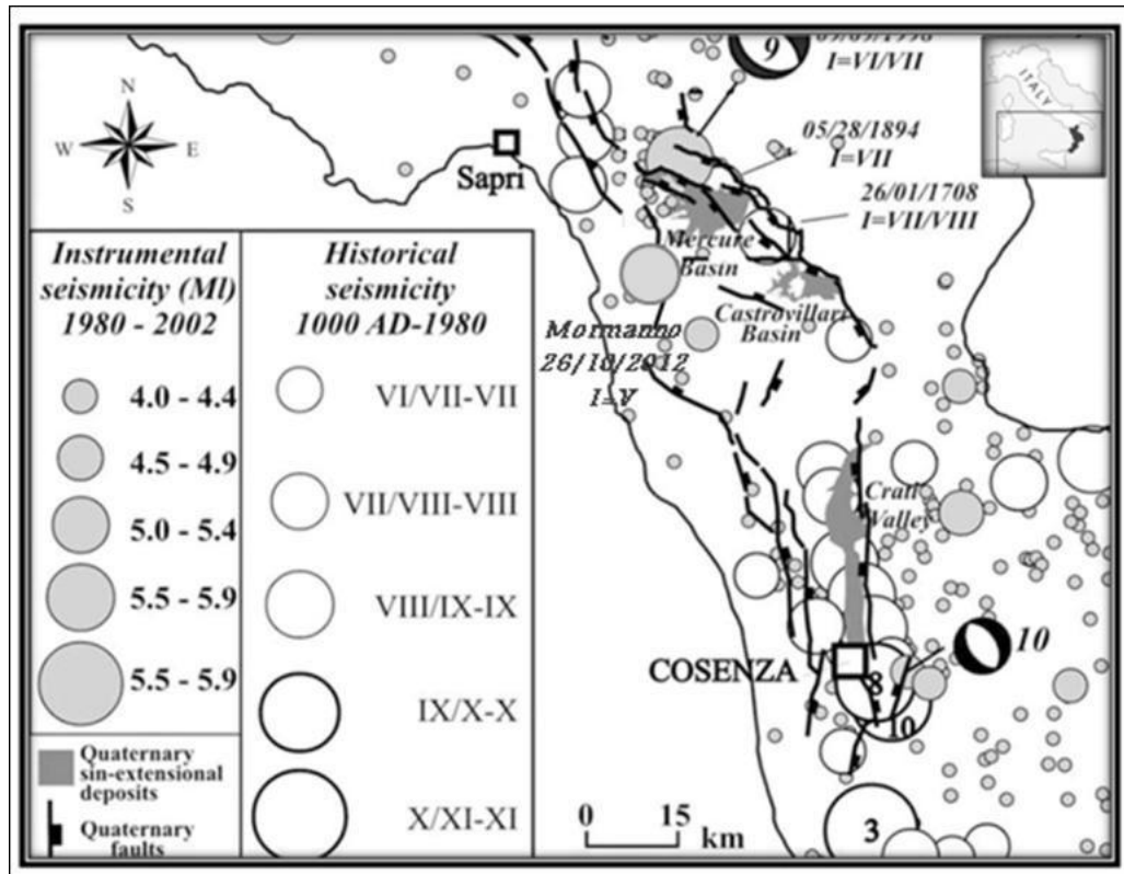
Figura 337. Maggiori faglie e sismicità nell'area del Pollino e nella parte settentrionale della Calabria. Da: Brozzetti et al., 2009.
