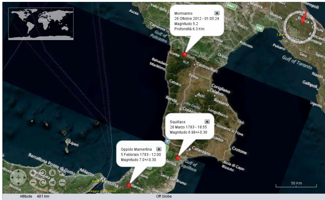
Figura 389. Posizioni e dati relativi alle scosse di magnitudo maggiore relative ai terremoti del Pollino del 2012 e della Calabria meridionale del 1783.
